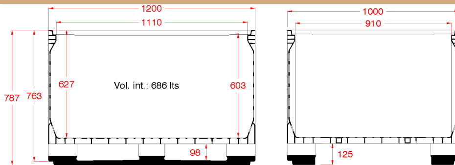
Palox 1200 x 1000 x 787 mm., fond et parois pleins, 2 semelles
